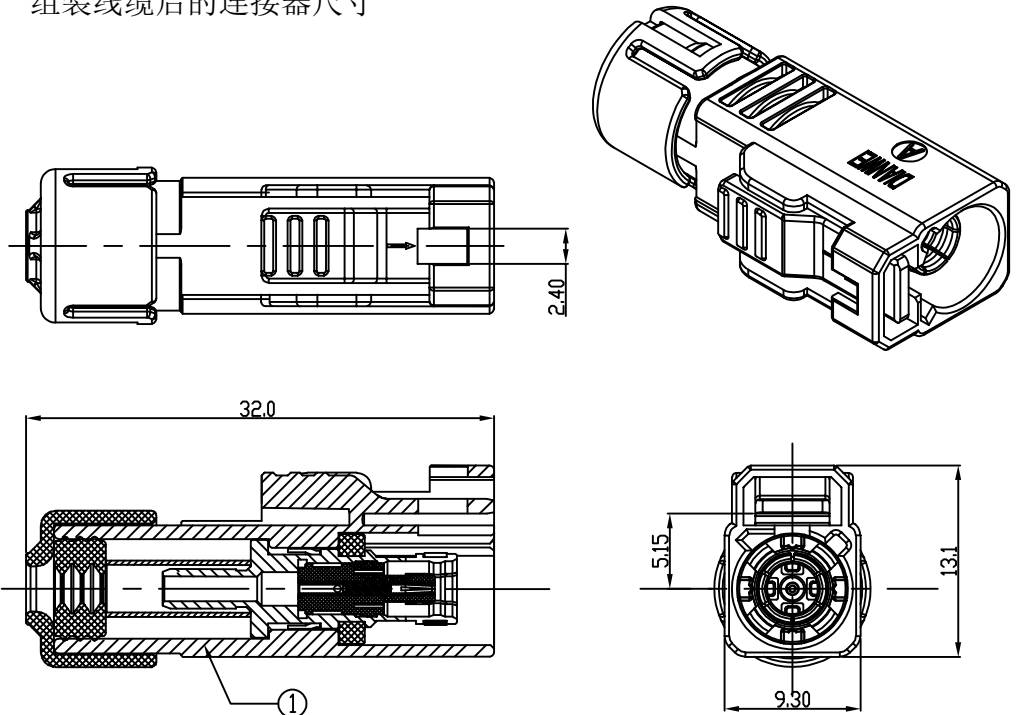
组装线缆后的连接器尺寸
